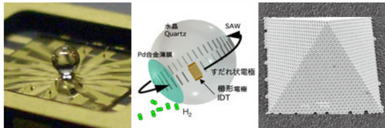
水晶の球を用いた高性能の水素ガスセンサ ボール SAW 水素ガスセンサの構造と原理 マイクロ粒子を自己配列によって面立方格子に並べたもの
